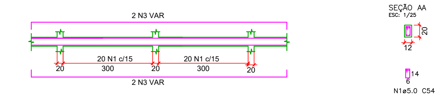
DETALHE - VIGAS BALDRAME S/ ESCALA Perímetro: 369,59 metros lineares
